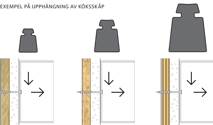
SPÅNSKIVA ELLER MEDELHÅRD TRÄFIBERSKIVA OCH GIPSSKIVA OSB-SKIVA OCH GIPSSKIVA PLYWOOD ELLER TRÄFIBERSKIVA AV KONSTRUKTIONSKVALITET OCH GIPSSKIVA
