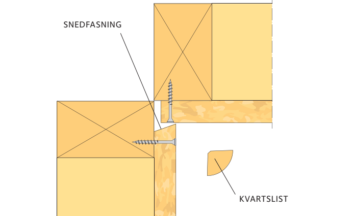
SNEDFASNING AV KANTEN PÅ SISTA SKIVAN UNDERLÄTTAR MONTERINGEN. EN KVARTSLIST TÄCKER SKRUVARNA I HÖRNET.
