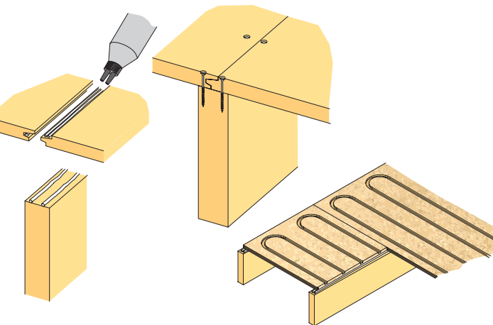
NOT- OCH FJÄDERLIMNING AV GOLVSPÅNSKIVOR MED SKRUV OCH DUBBELPIPIG LIMFLASKA GOLVSPÅNSKIVOR MED SPÅR FÖR VATTENBUREN GOLVVÄRME
